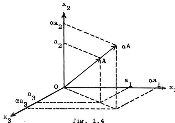
Het produkt van een 3-dimensionale vector A en een reëel getal \alpha
